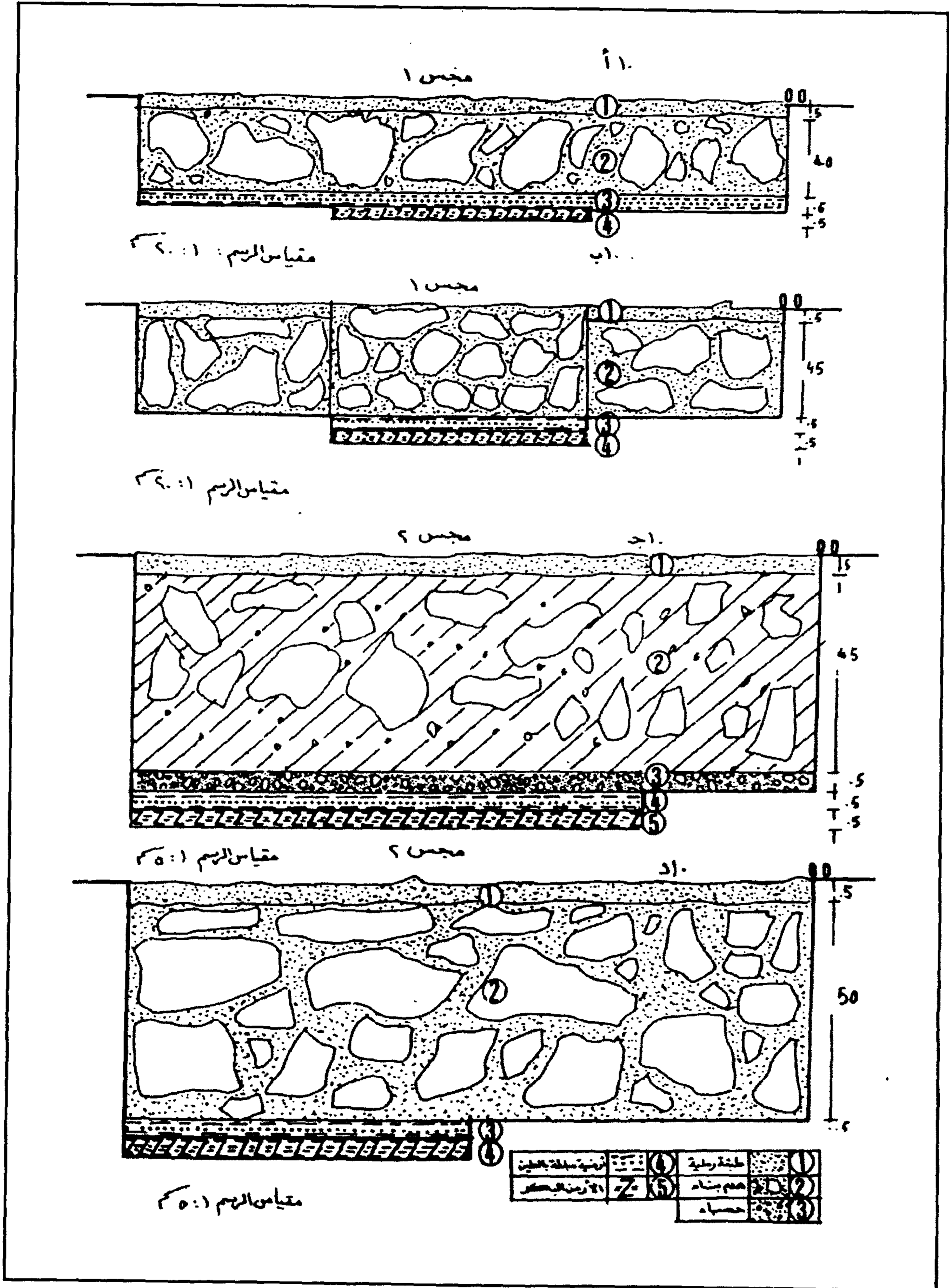
لوحة ١٠: رسم يوضح تراكيب الطبقات في المجسنة .
